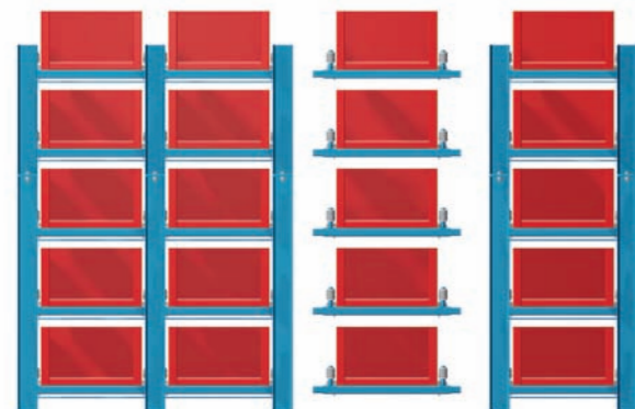
Grundgestell mit zwei Feldern / Verbindungsfeld / Grundgestell mit einem Feld
